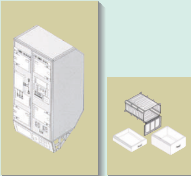
実験装置が組み込まれるラック（左）とロッカー（右） Rack (left) and locker (right) accommodate the experimental units
