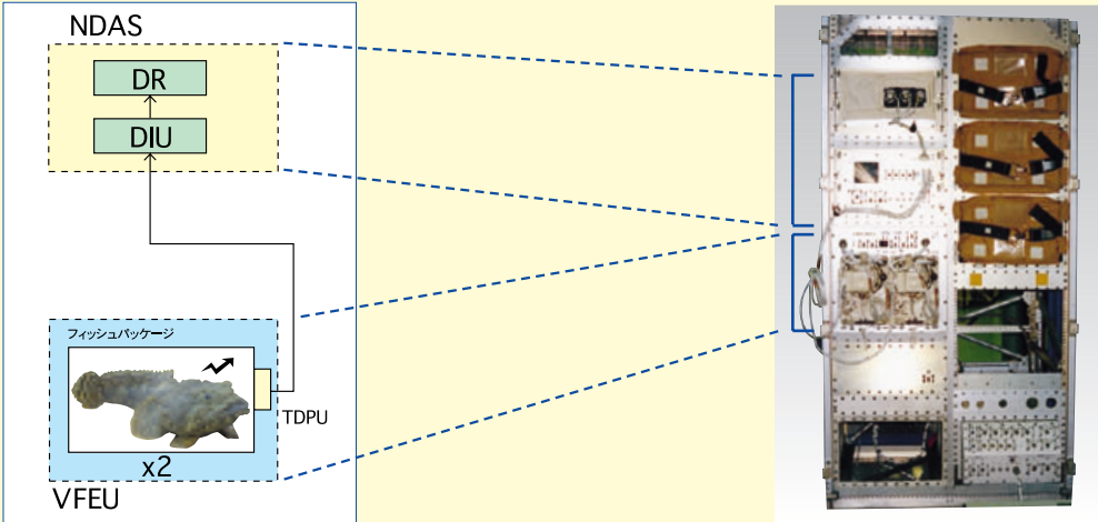
スペースハブ・ラックに組み込まれたVFEU / NDAS VFEU / NDAS installed in SPACEHAB Rack
