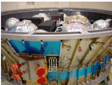
Fig. 1.2.5-1 Propulsion Module
