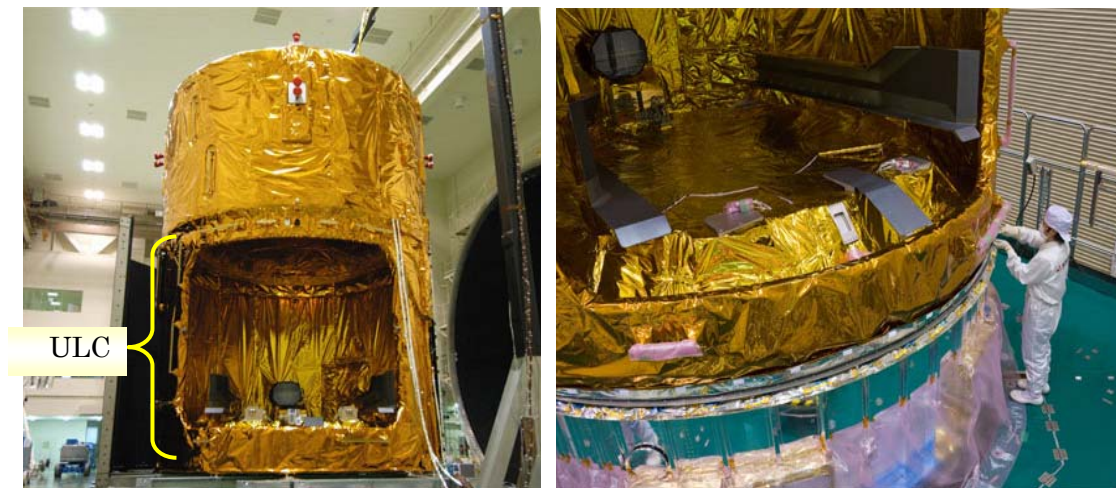
Fig. 1.2.2-1 ULC (HTV-1)
