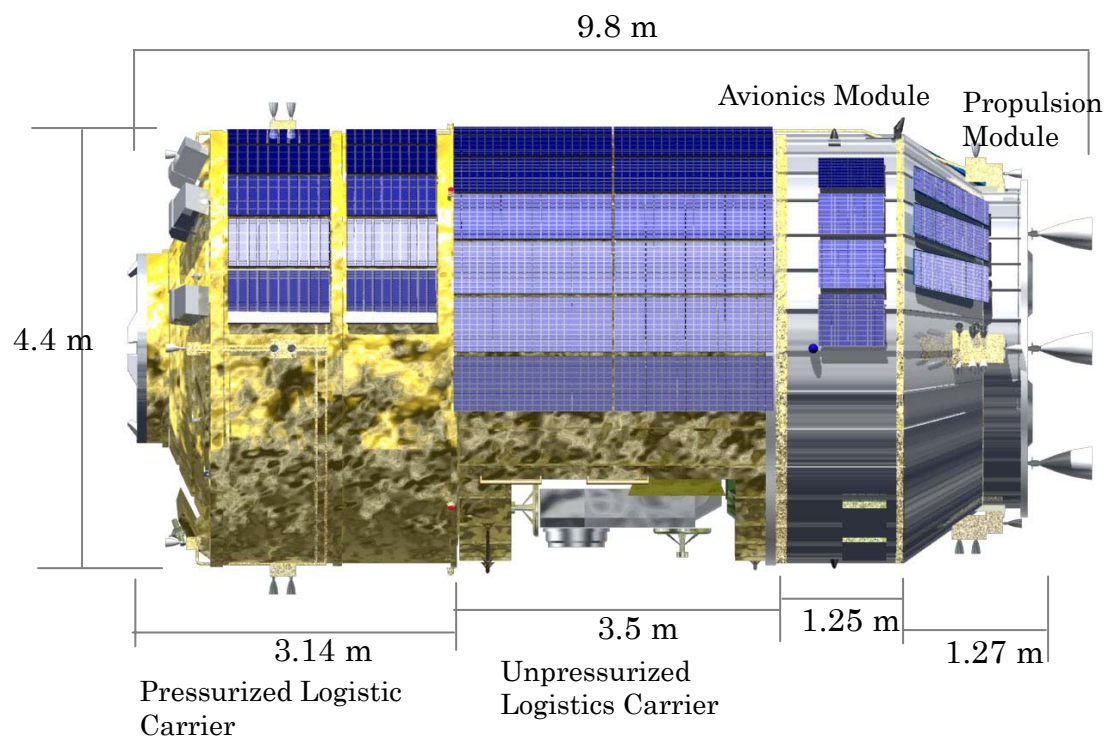
Fig. 1.2-2 HTV Dimensions
