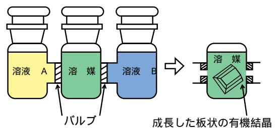
有機結晶成長実験装置 (OCC) Organic Crystal growth Chamber
