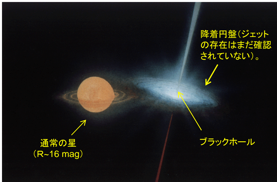
ブラックホール候補天体 XTE J1752-223 の想像図
