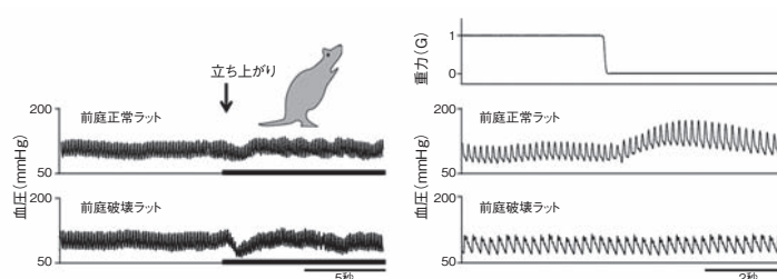
図1 立ち上がり(左図)、および自由落下による微小重力(右図)に対する血圧応答
