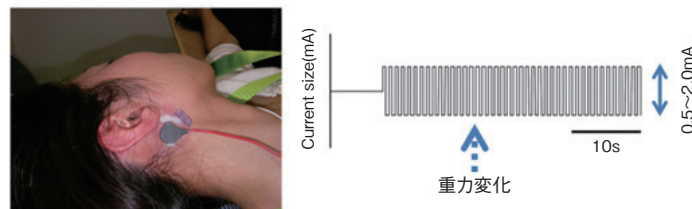
図2 耳の後ろに置いた1対の刺激電極を用いて、体表上から前庭を電気刺激
