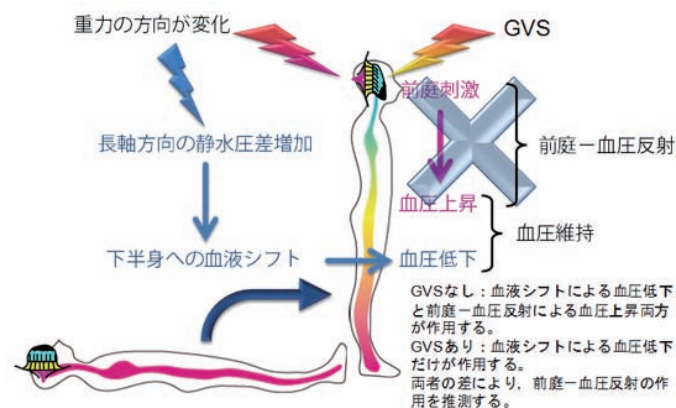
図3 GVSにより姿勢変化による前庭系入力をマスクして、前庭—血圧反射による血圧調節をブロックし、前庭—血圧反射の作用を推測する仕組み
