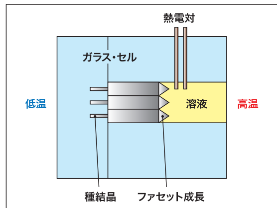
図5 結晶成長実験に使う試料容器の断面図
