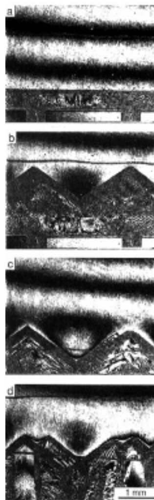
図2 時間とともにファセット成長するザロール結晶(地上) (干渉縞画像:時間経過は(a)→(b)→(c)→(d))
