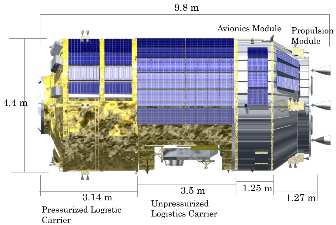
Fig. 1.2-2 HTV Dimensions
