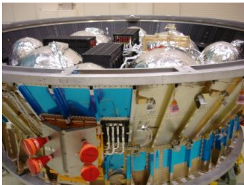
Fig. 1.2.5-1 Propulsion Module
